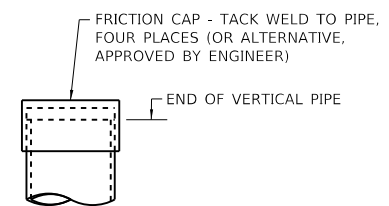
FRICION CAP DETAIL
